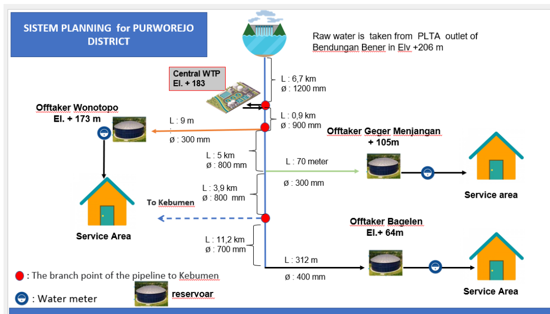
Gambar 2.98 System Planning Bendungan Bener di Kabupaten Purworejo
