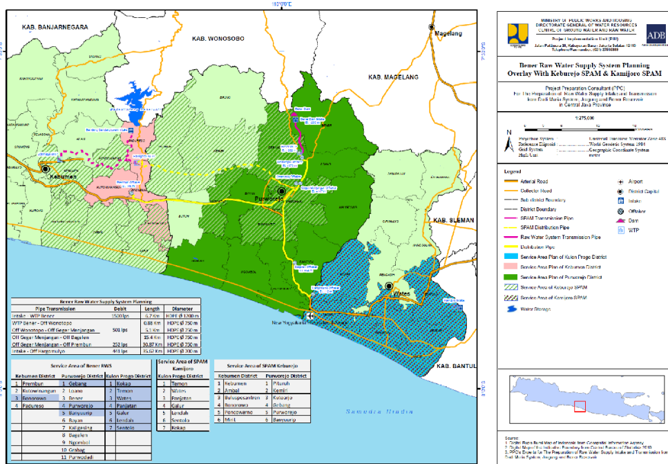
Gambar 2.99 Raw Water Supply Bendungan Bener dengan SPAM Regional Keburejo dan SPAM Regional Kamijoro
