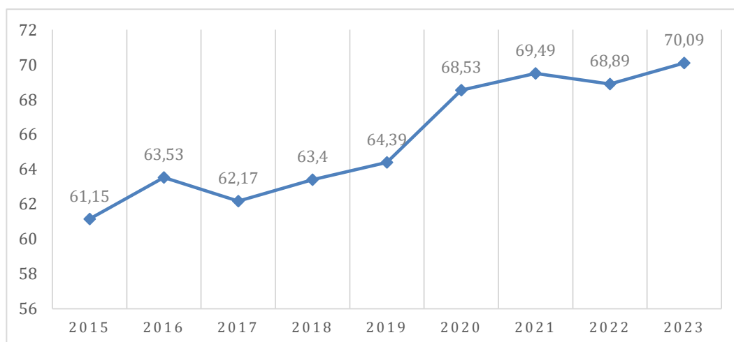
Gambar 2.94 Capaian Indeks Kinerja Sistem Irigasi (IKSI) Kabupaten Purworejo Tahun 2015-2023
